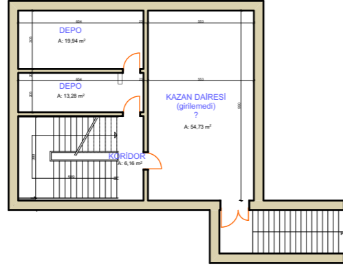
FEN FAKÜLTESİ C BLOK BODRUM KAT PLANI
