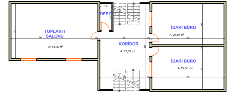
FEN FAKÜLTESİ F BLOK ZEMİN(+1.50 KOTU) KAT PLANI
